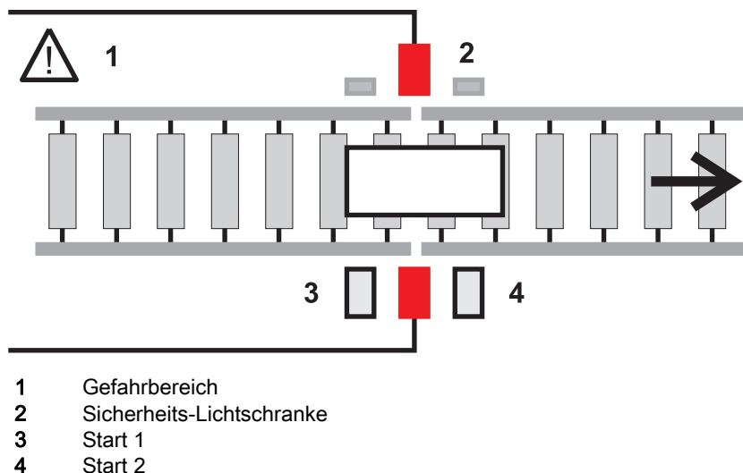
Bild 3.4: Phase 4 - Fortsetzung des Muting-Prozesses mit der Belegung von Start 2 durch die Palette.
