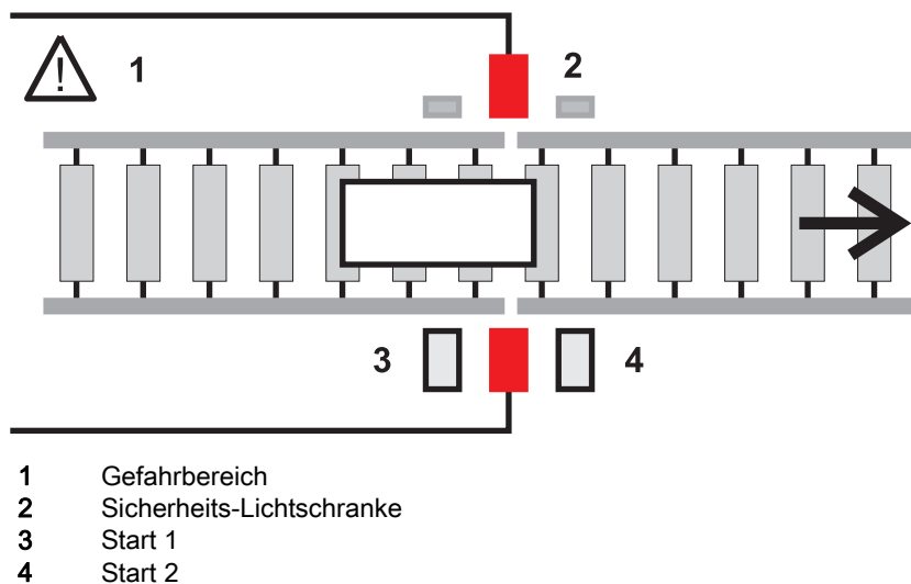
Bild 3.3: Phase 3 - Sicherheits-Lichtschanke wird unterbrochen.
