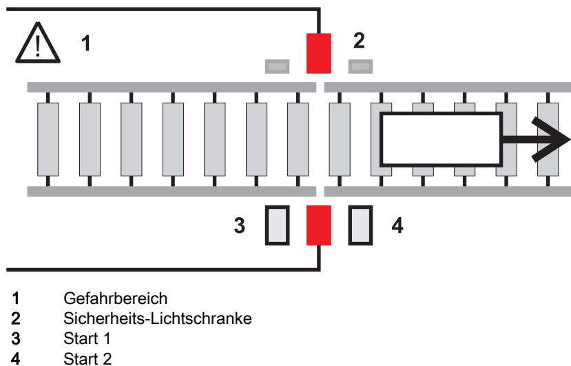
Bild 3.7: Phase 7 - Muting beenden
