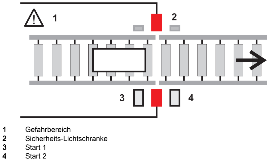
Bild 3.2: Phase 2 - Muting wird durch Unterbrechung von Start 1 aktiviert.
