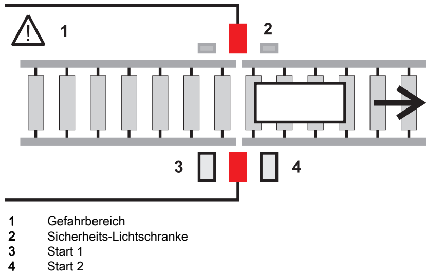
Bild 3.6: Phase 6 - Sicherheits-Lichtschanke wird wieder frei.
