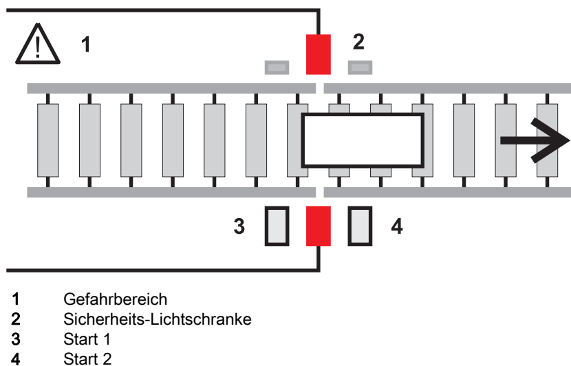
Bild 3.5: Phase 5 - Muting dauert auch nach dem frei werden von Start 1 an.
